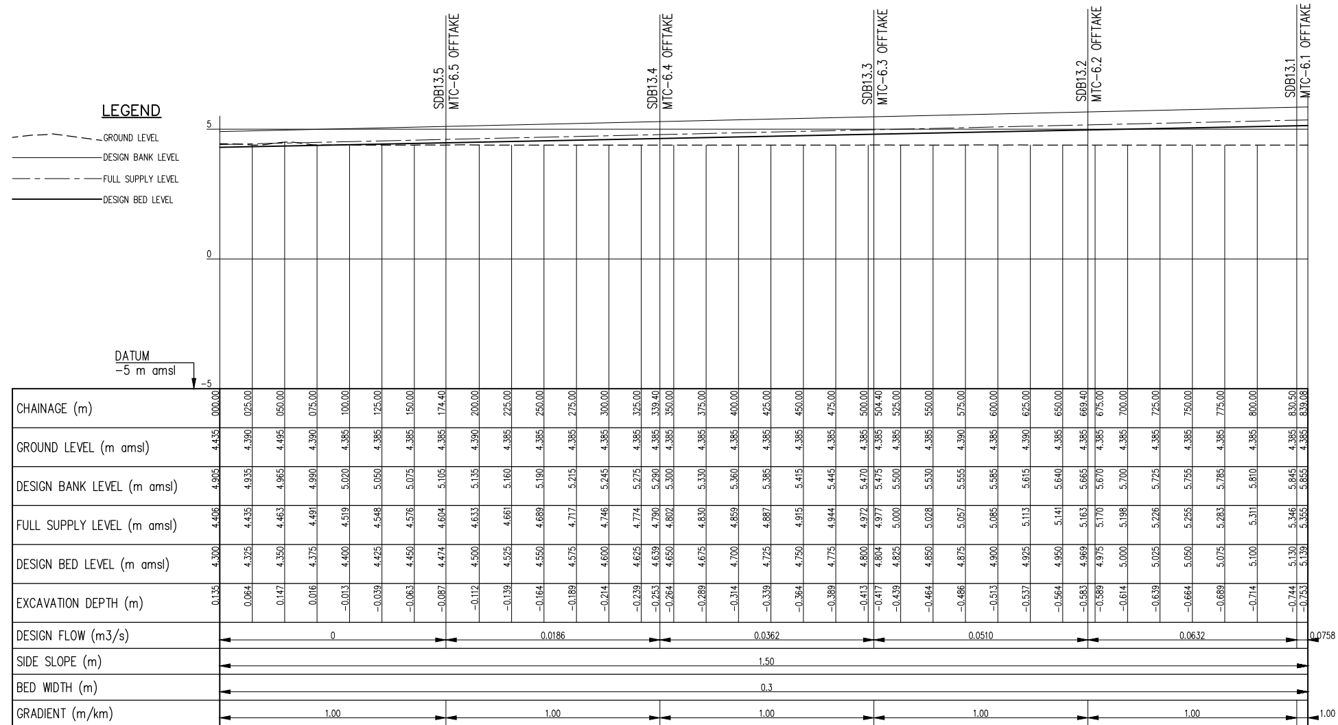
MSC-6 PROFILE SCALE: Hor 1:2000, Ver 1:100
