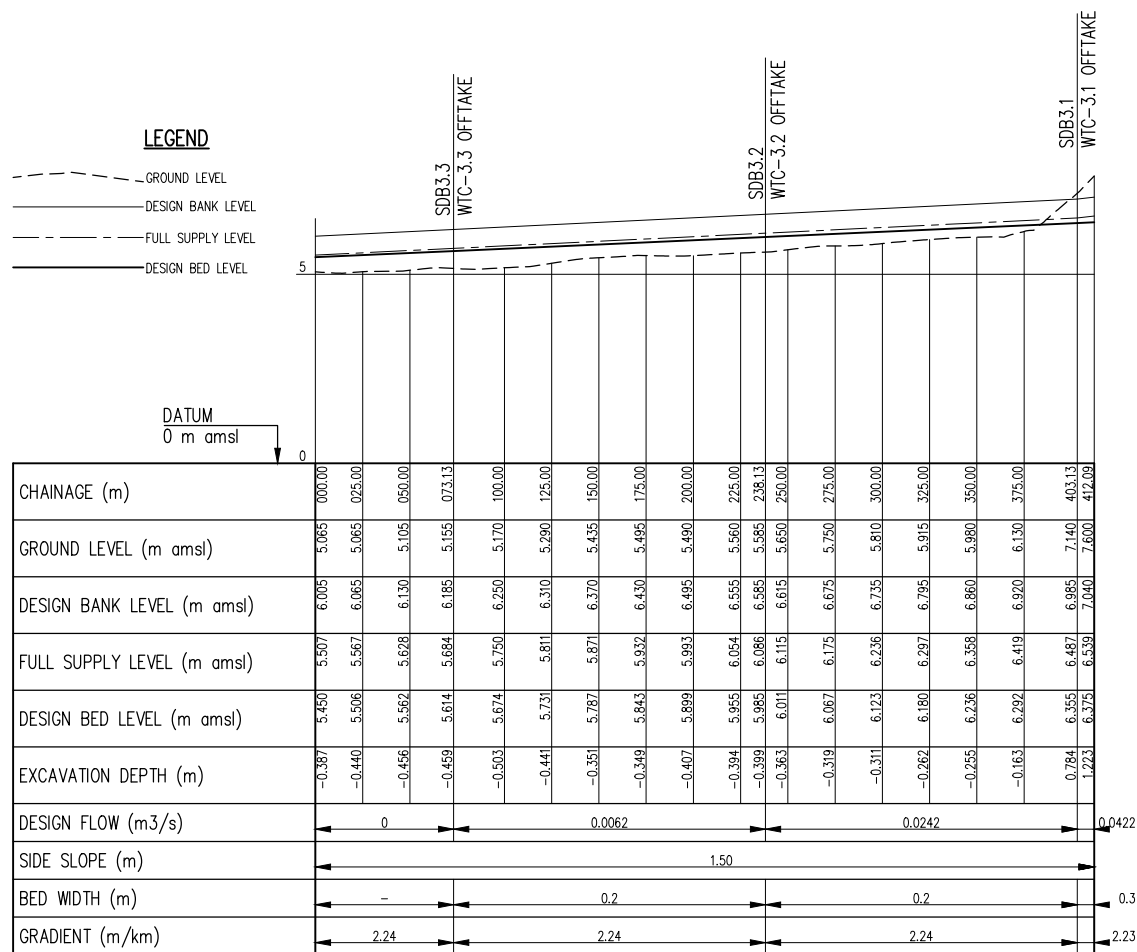
WSC-3 PROFILE SCALE: Hor 1:2000, Ver 1:100
