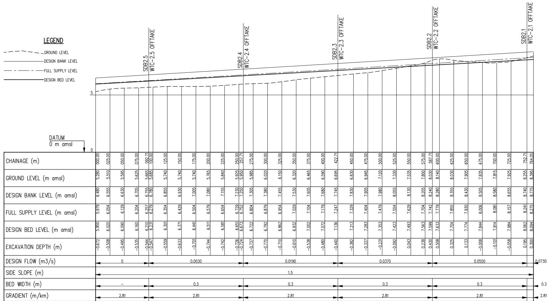
WSC-2 PROFILE SCALE: Hor 1:2000, Ver 1:100
