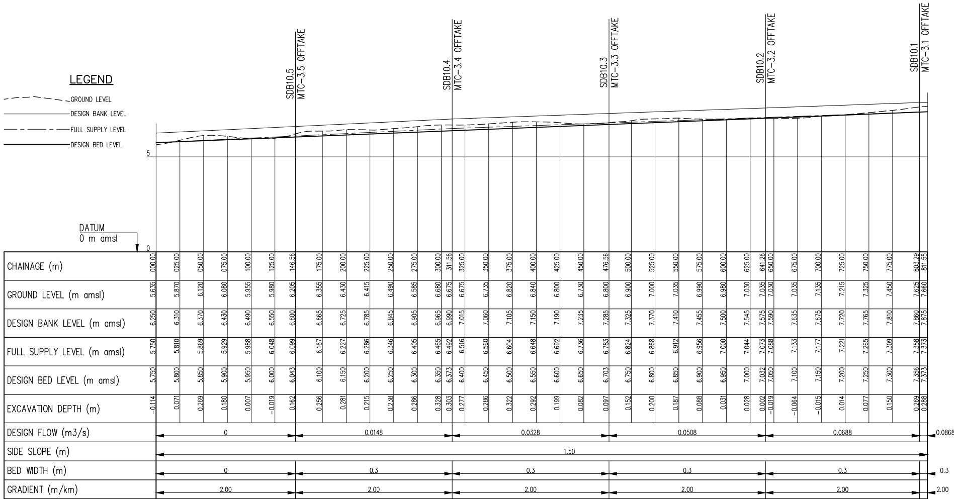
MSC-3 PROFILE SCALE: Hor 1:2000, Ver 1:100
