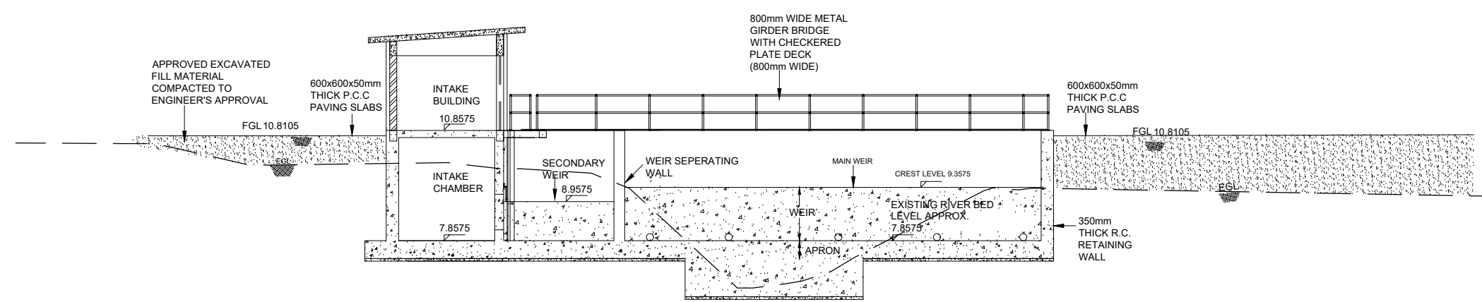
SECTION A-A
