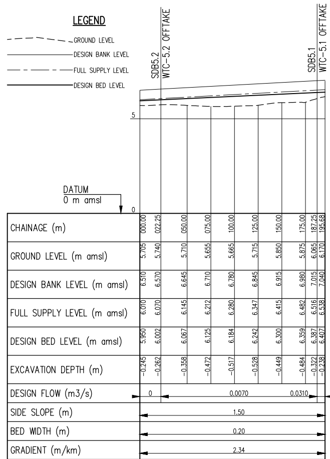
WSC-5 PROFILE SCALE: Hor 1:2000, Ver 1:100
