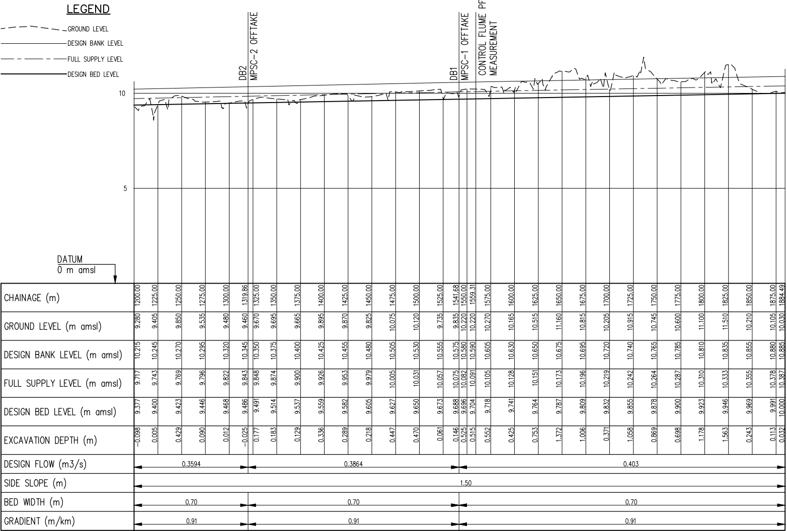
MPMC PROFILE SCALE: Hor 1:2000, Ver 1:100
