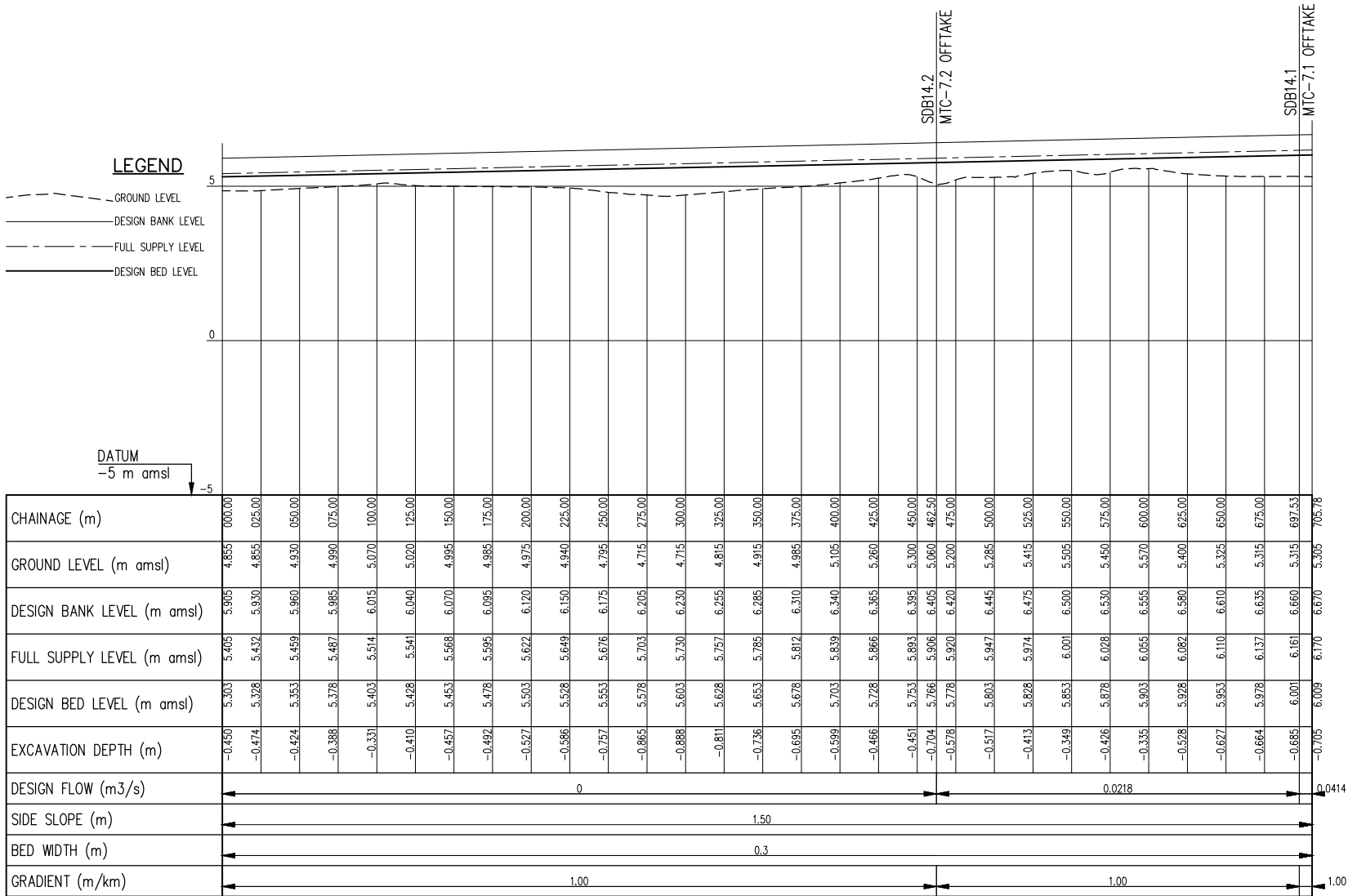
MSC-7 PROFILE SCALE: Hor 1:2000, Ver 1:100
