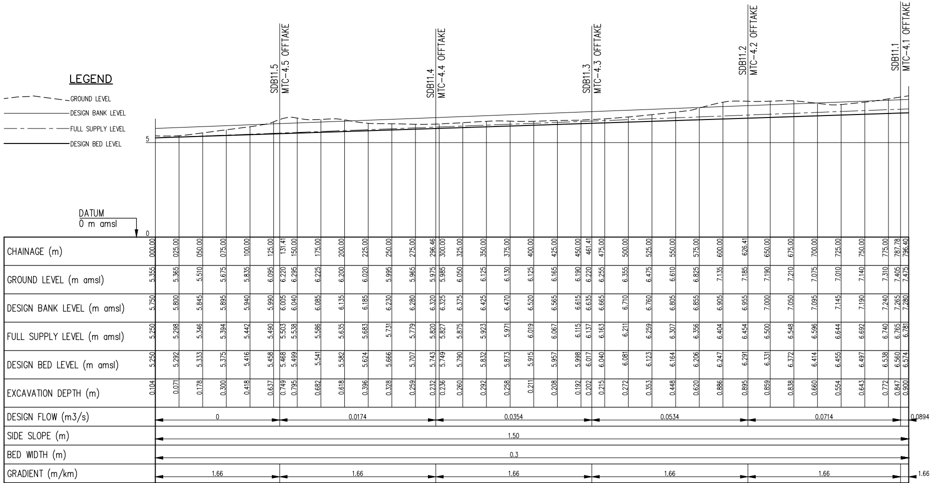
MSC-4 PROFILE SCALE: Hor 1:2000, Ver 1:100
