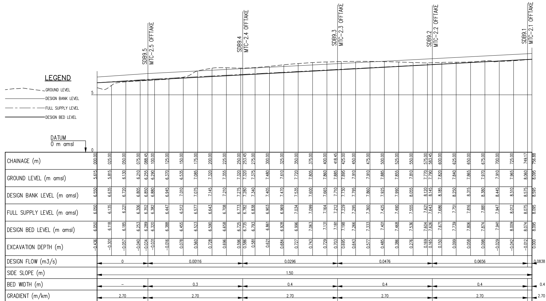
MSC-2 PROFILE SCALE: Hor 1:2000, Ver 1:100
