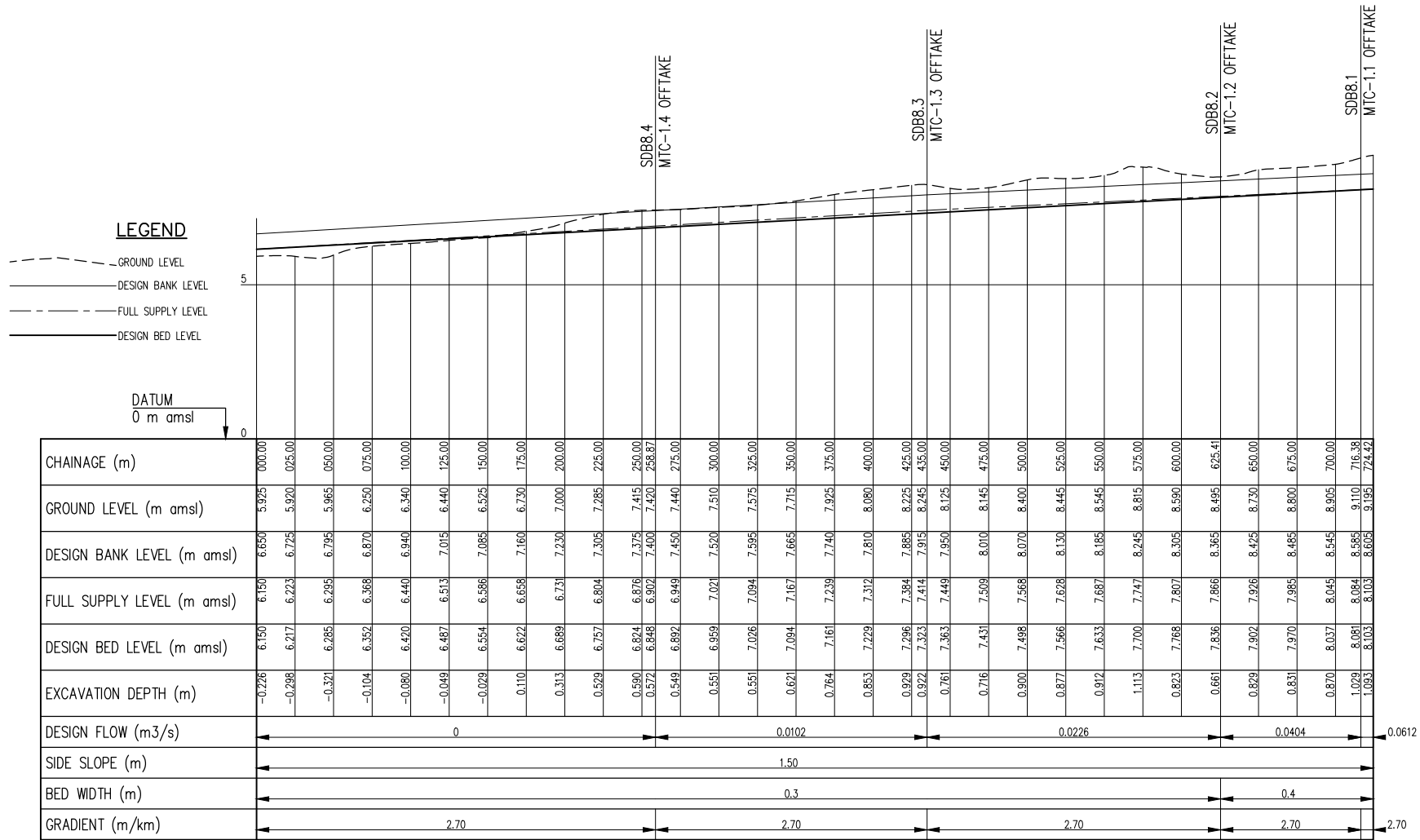
MSC-1 PROFILE SCALE: Hor 1:2000, Ver 1:100
